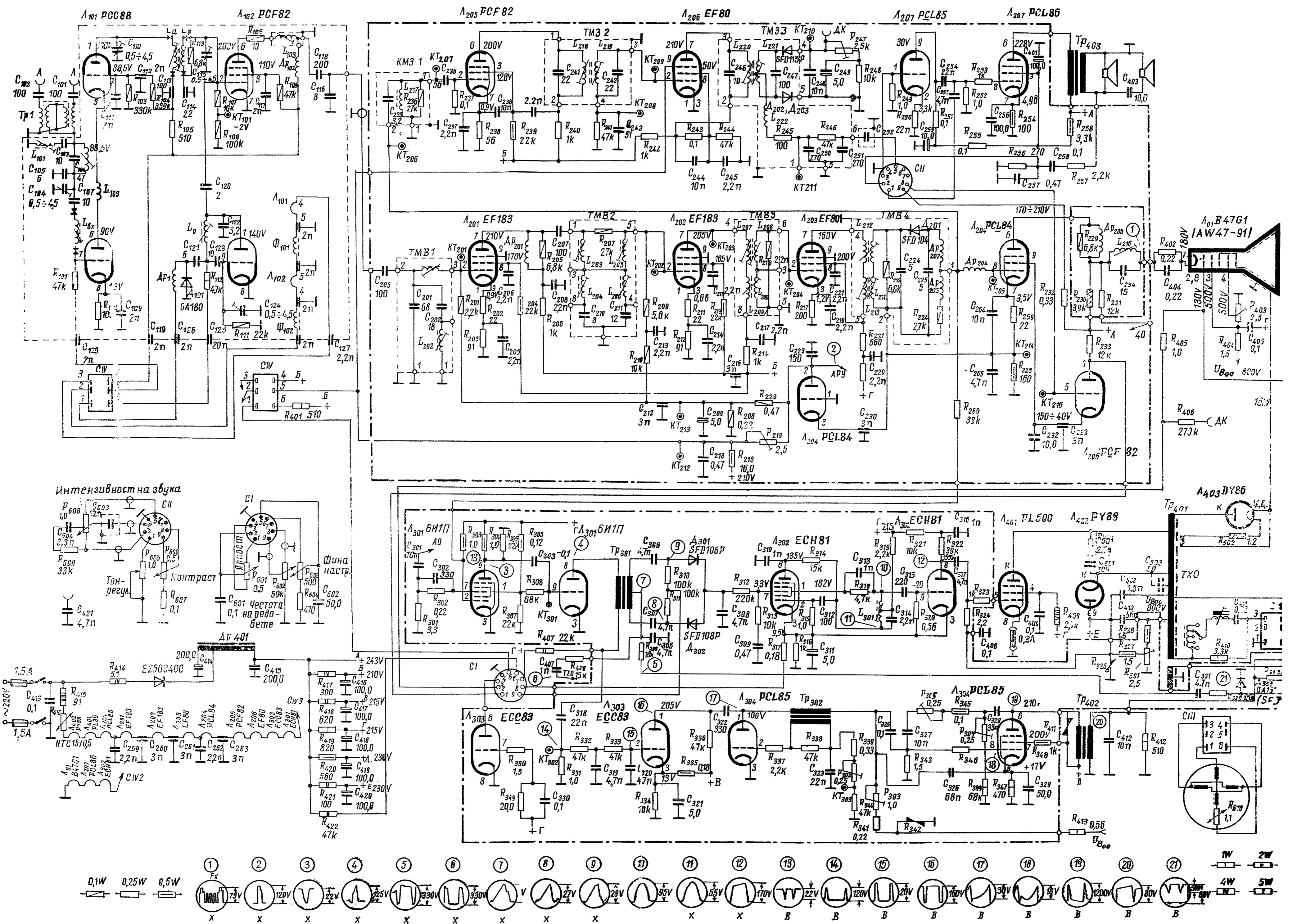
Приложение 1. Схема на телевизора "ПИРИН"
